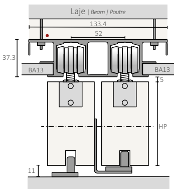
Porta de madeira Wooden door | Porte en bois
