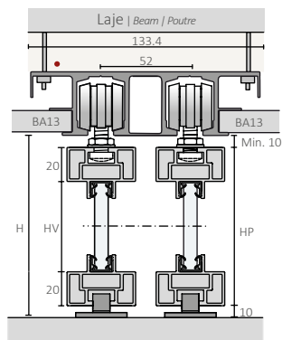
Porta de vidro com moldura em alumínio Dimensão máxima 1200x2600mm
